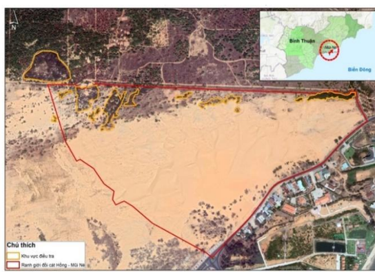
Hình 1. Sơ đồ vị trí điều tra thực vật ở khu vực Đồi Hồng, Mũi Né, thành phố Phan Thiết, tỉnh Bình Thuận
